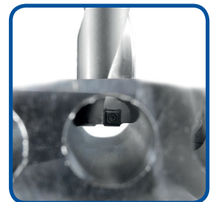
Çoklu delik delme Cross-hole drilling
